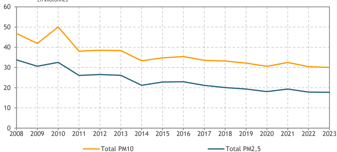
Graphique 4 Évolution des émissions de \text{PM}_{10} et \text{PM}_{2,5} entre 2008 et 2023 En kilotonnes
